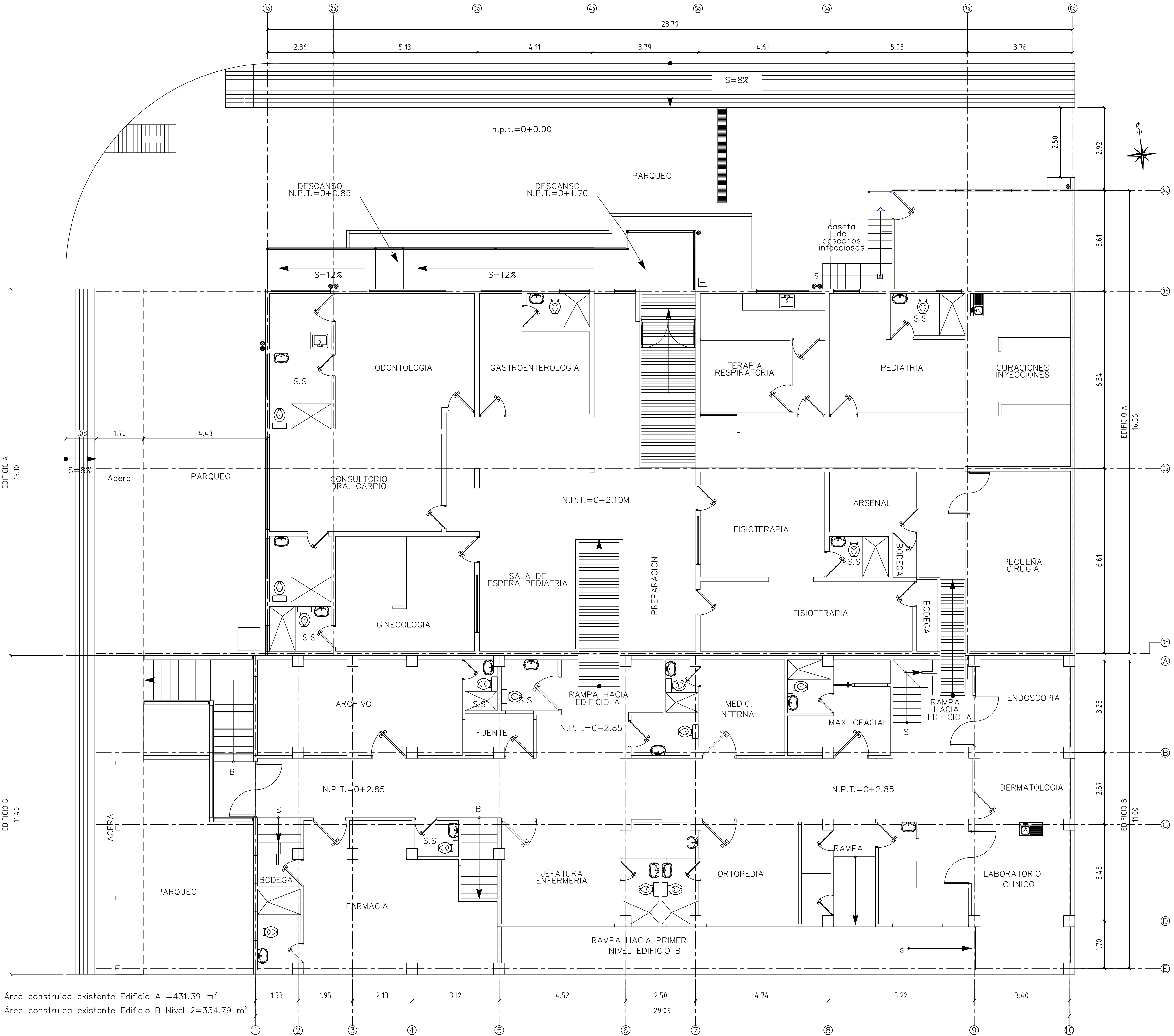
PLANTA ARQUITECTONICA EDIFICIO B 2° NIVEL
